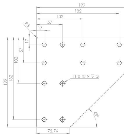
L-Verbindung 80mm
