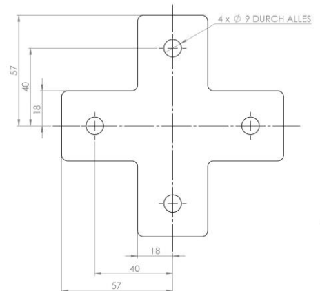
Kreuzverbindungsbleche
