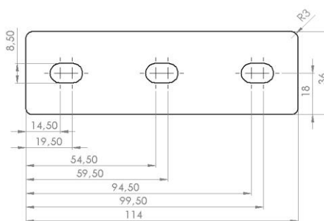
Verbindungsbleche 114mm
