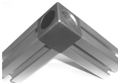
Würfelerbinder 2D für 2 Profile
