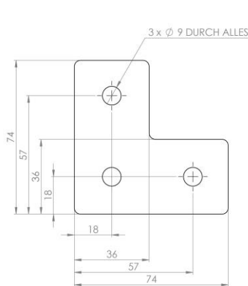
L-Verbindungsbleche
